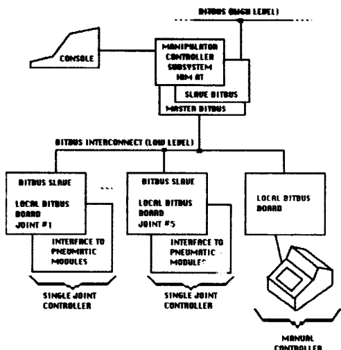
Fig. 4. Manipulator controller.
